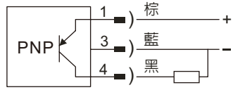
圖7 PNP輸出型
