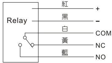
圖8 5A 繼電器輸出型
