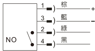
圖9 1A 繼電器輸出型(NO)
