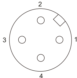
圖12 連接器腳位圖 (NPN & PNP 輸出型及1A繼電器輸出型)
