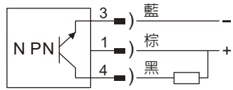
圖6 NPN輸出型
