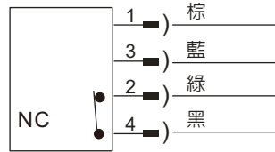
圖10 1A 繼電器輸出型(NC)
